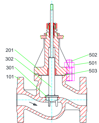
MV 5311, PV 6311 DN 65 – 150, PN 63 – 160
