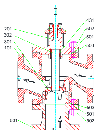
MV 5321, PV 6321 DN 100 – 150, PN 16 – 40
